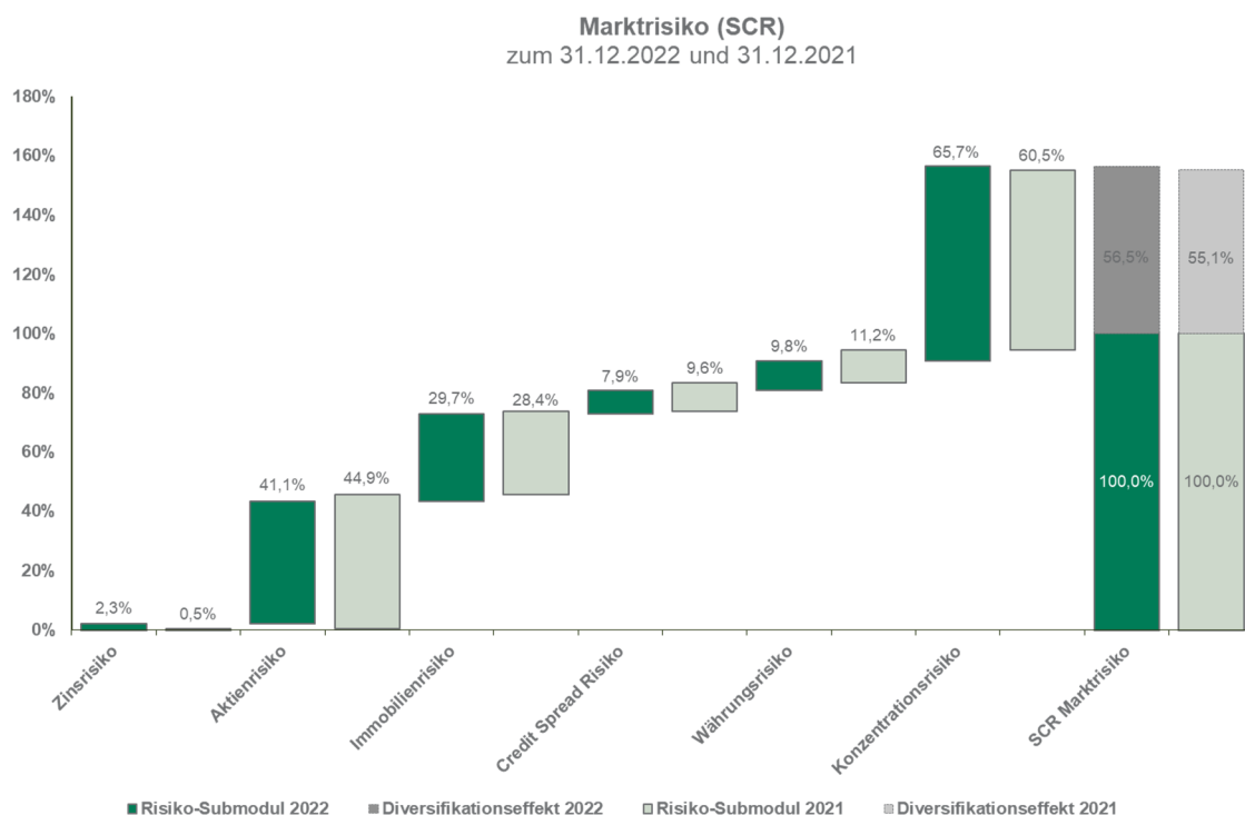
Abbildung 13: Marktrisiko
