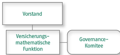
Abbildung 9: Versicherungsmathematische Funktion
