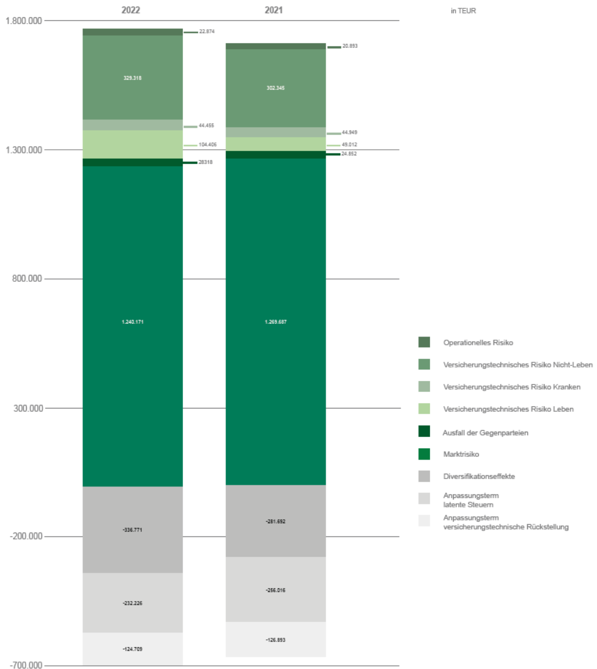
Abbildung 15: SCR Gesamt
