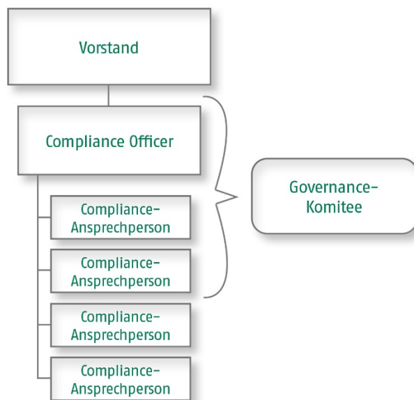
Abbildung 7: Compliance-Funktion
