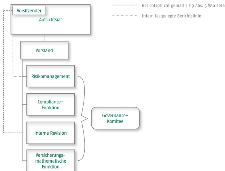
Abbildung 4: Organisatorische Eingliederung
